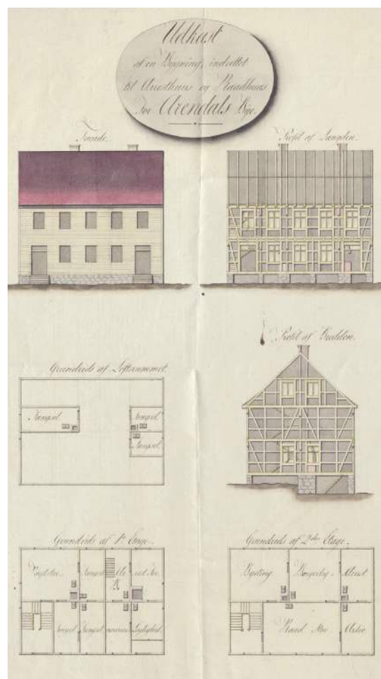
Grunntegning av arresthuset byfogd Berg foreslo å bygge på toppen av Tyholmen i august 1803. Foto: Riksarkivet.
